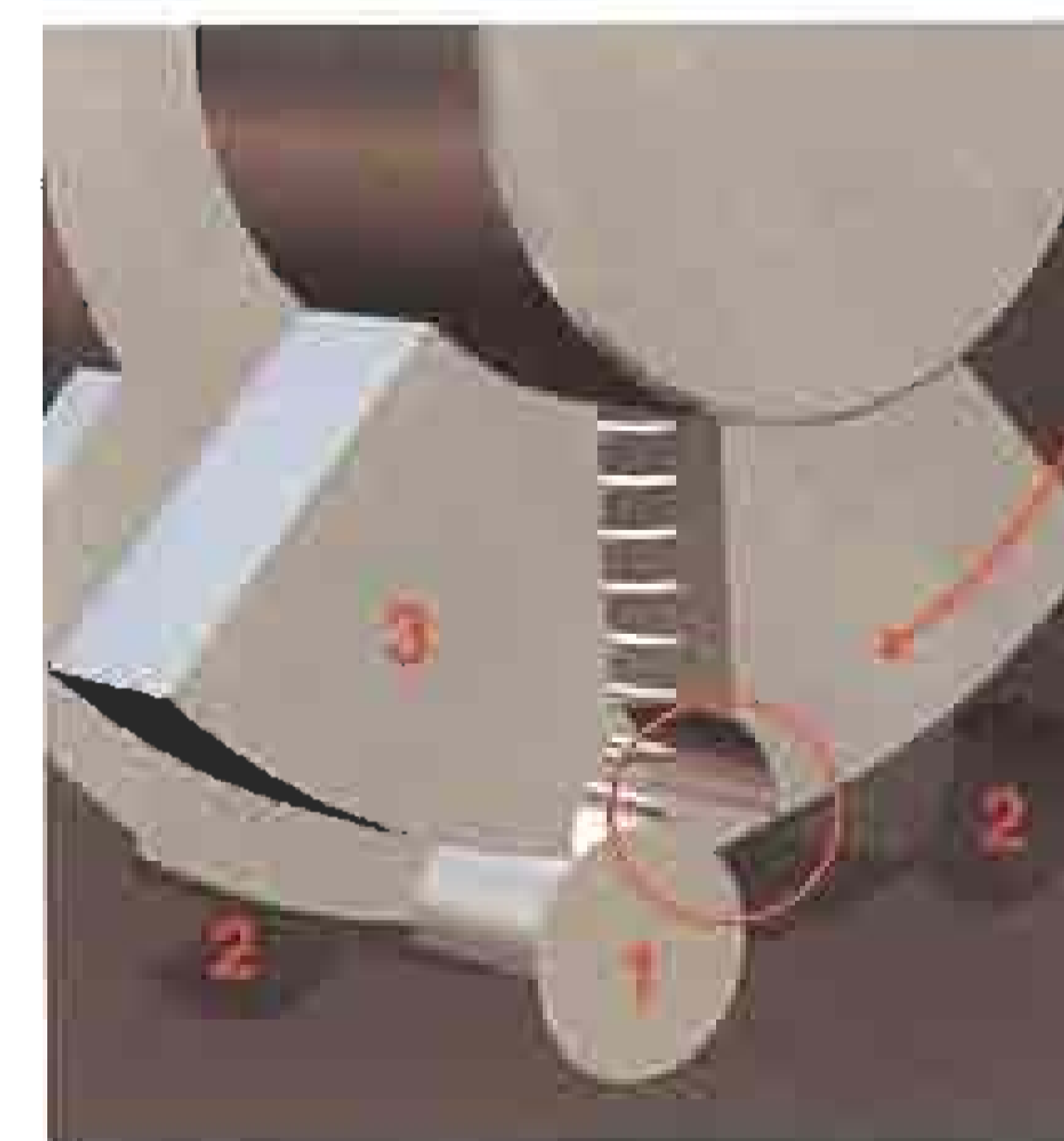
Při pokusu o vloupání jsou zajišťovací kolíky ① spojovacím prvkem ③ zatlačeny do drážek v pouzdře ②.
