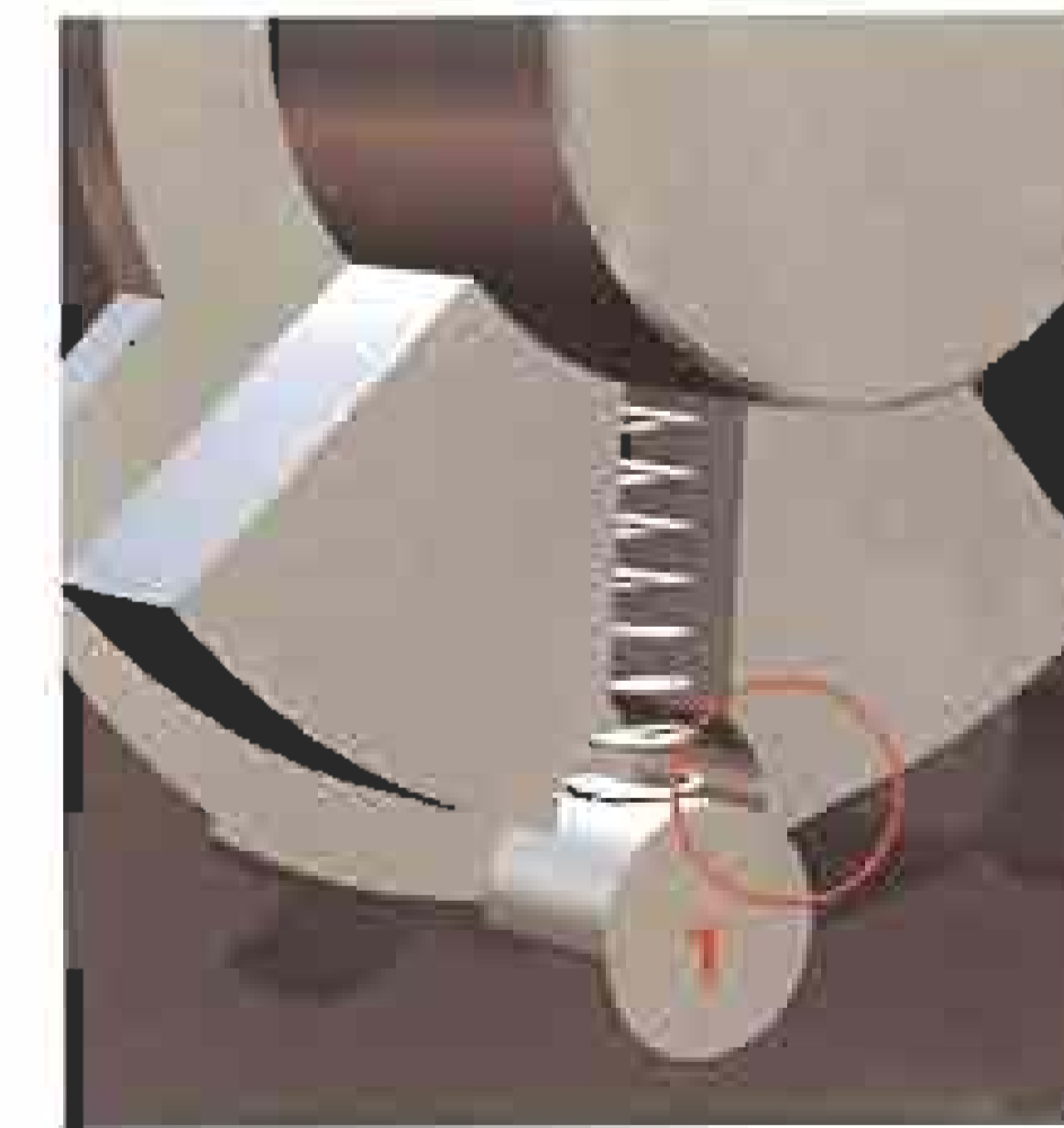
V této poloze kolíky ① účinně brání v otočení okenní kliky z venku. Okenní klička se zablokuje a zmaří pokus o vloupání.
