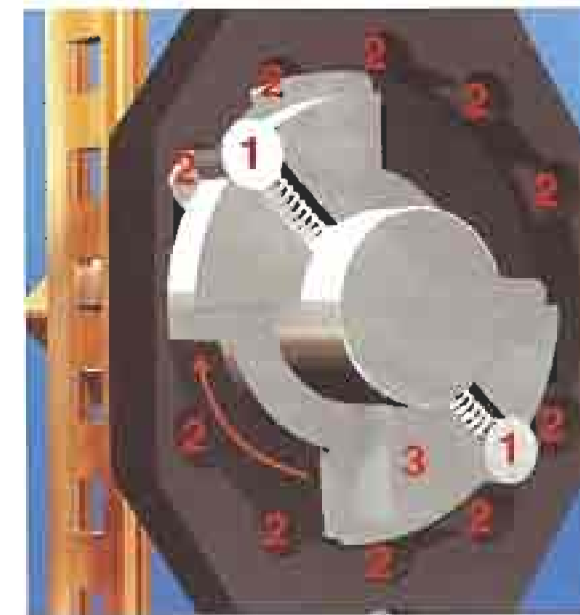
Během otáčivého pohybu jsou zajišťovací kolíky ① pomocí spojovacího prvku ③ unášeny k dalším drážkám ②, do kterých opět slyšitelně zapadnou.
