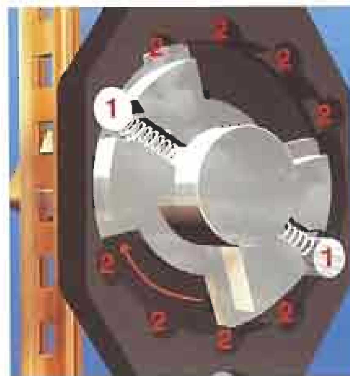
Při otáčení okenní klikou zapadávají pružně uložené zajišťovací kolíky ① přesným cvaknutím do speciálních drážek v pouzdře ② – tím vzniká typický zvuk Secustik® - slyšitelné plus pro větší bezpečnost.
