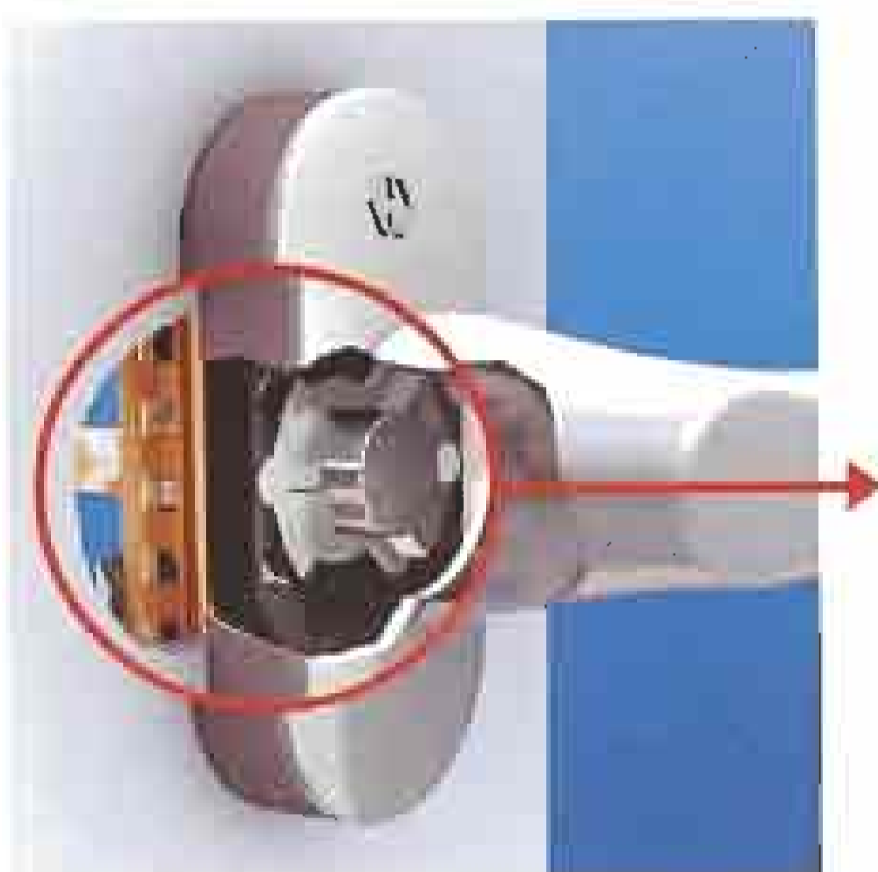
Patentovaný blokovací mechanismus okenní kliky Secustik®
